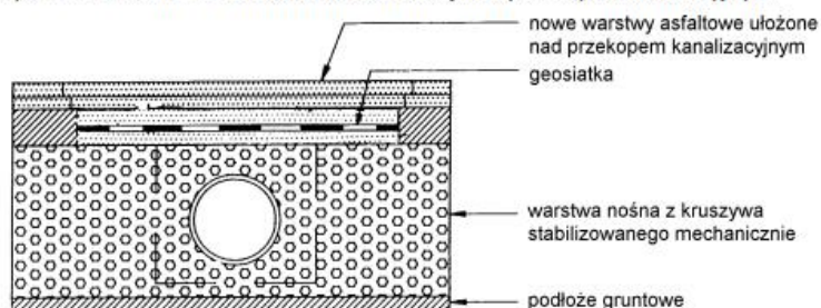
Rys. 1. Wzmocnienie nawierzchni asfaltowej nad przekopem instalacyjnym
