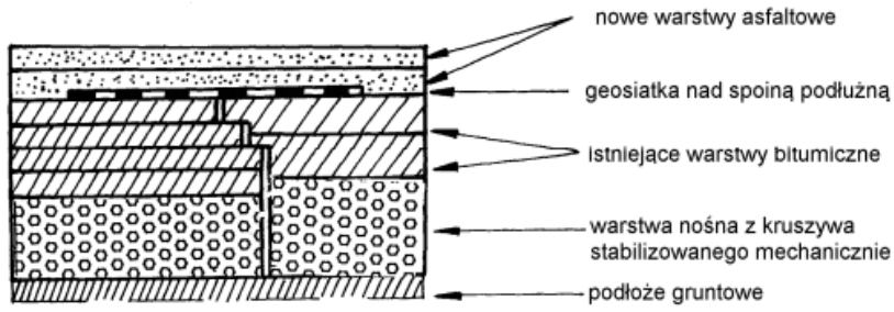
Rys. 5. Wzmocnienie nawierzchni asfaltowej w strefie poszerzenia nawierzchni
