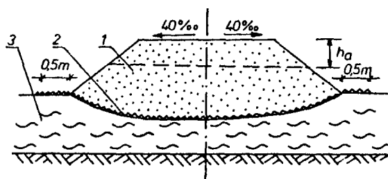
Rys. 2.1. Schemat nasypu na gruncie słabonośnym z zastosowaniem geosyntetyku 1 - nasyp drogowy, 2- warstwa geosyntetyki, 3 - grunt słabonośny
