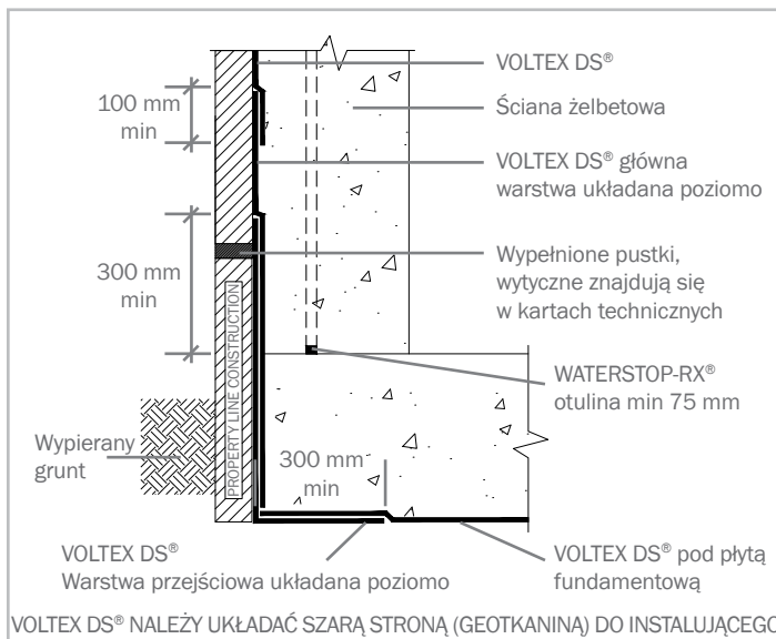
Przeście izolacji pionowej ze stałej obudowy wykopu na powierzchnię poziomą
