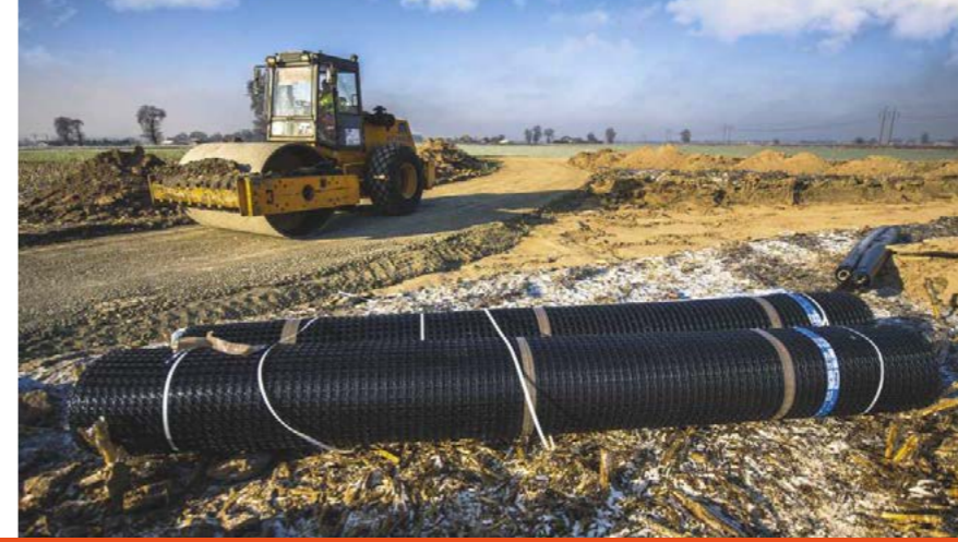
📍 Inczew (woj. łódzkie) 📄 Budowa dróg technologicznych i dojazdowych do farmy wiatrowej, placów montażowych oraz platform roboczych 🧺 Polgrid 30/30 180.000 m 2
