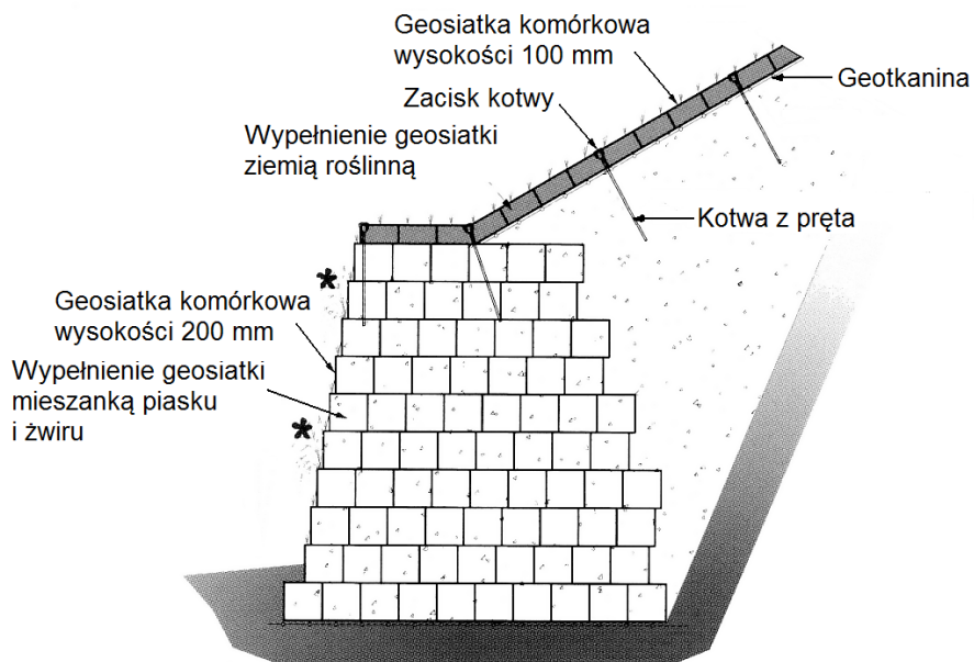
d) Przekrój poprzeczny niskiej ściany oporowej oraz umocnionej skarpy, wykonanych z geosiatki komórkowej
